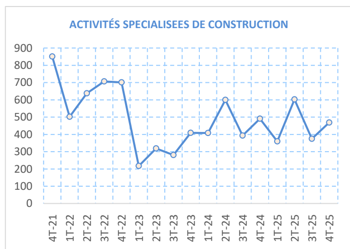
Figure 5 : ICA dans les activités spécialisées de construction
