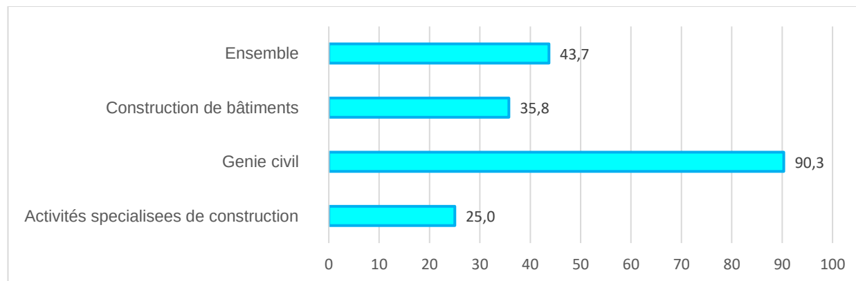
Figure 1 : Variation trimestrielle de l'Indice du chiffre d'affaires dans la Construction
