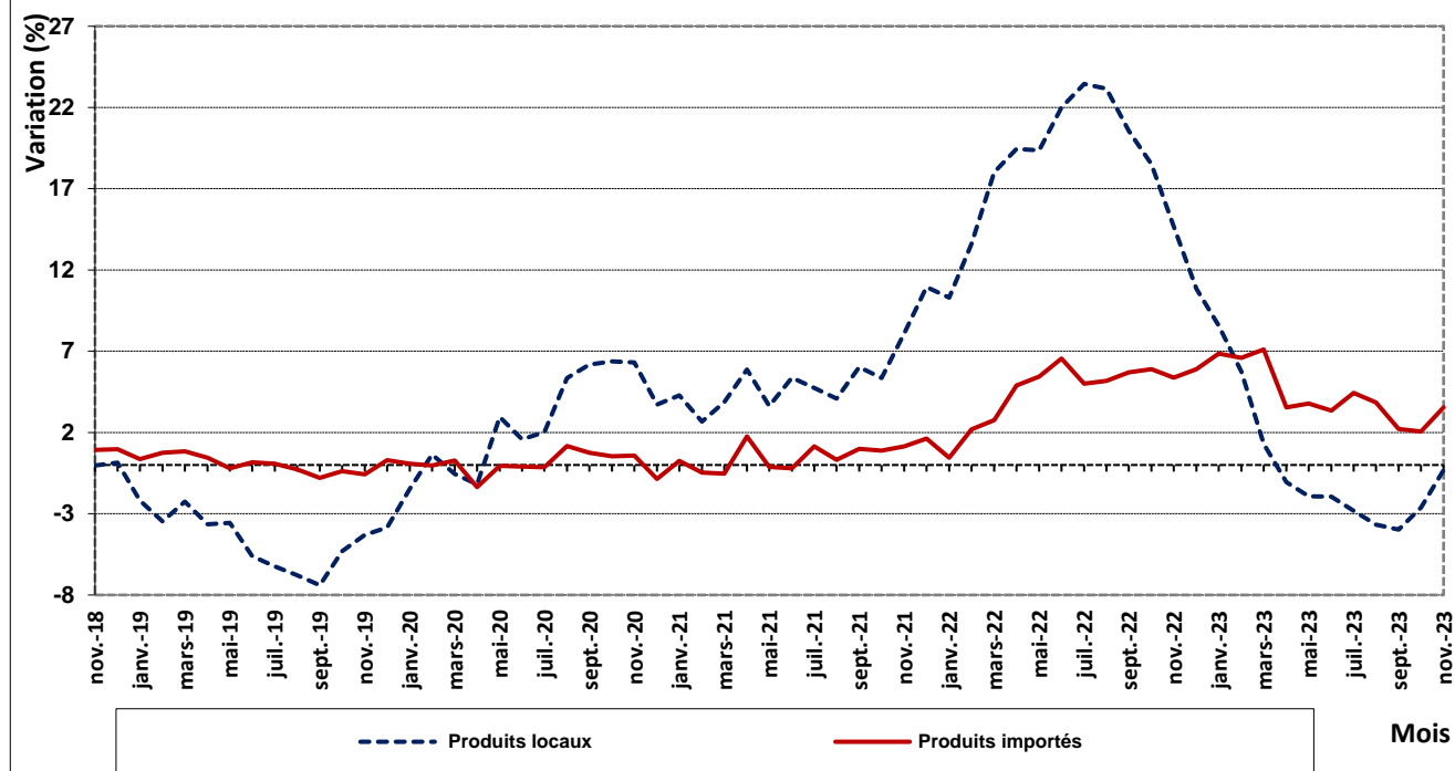
Graphique N°4: Glissement annuel des indices produits locaux et des indices produits importés
